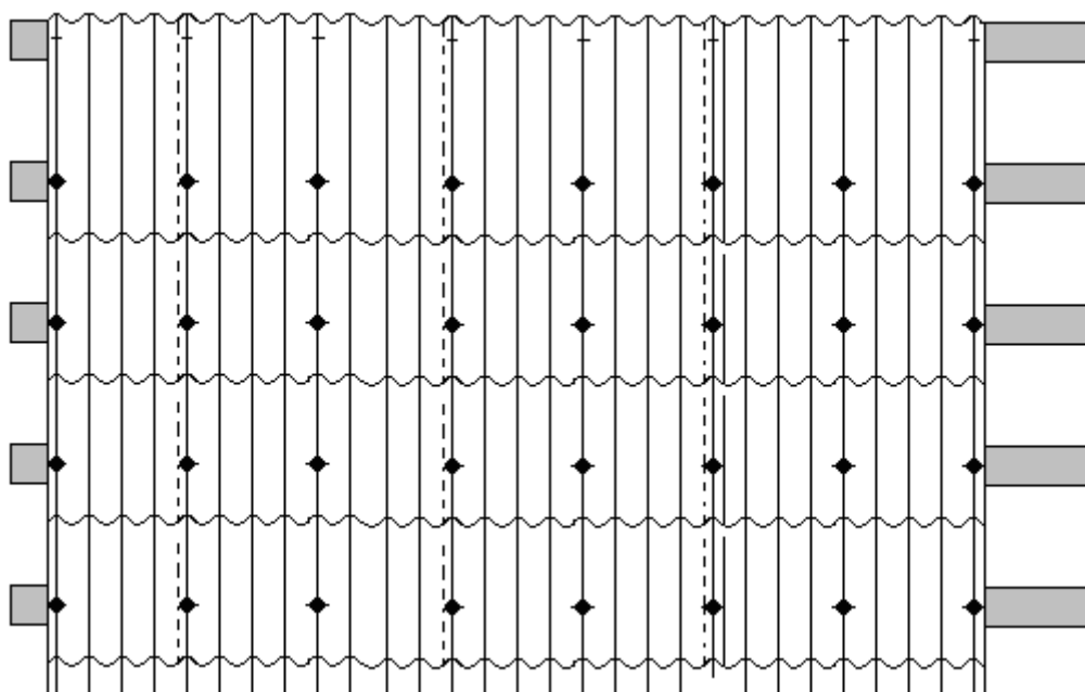
Рисунок 2. Схема монтажа и точки крепления черепицы Керамопласту при укладке листов без смещения
