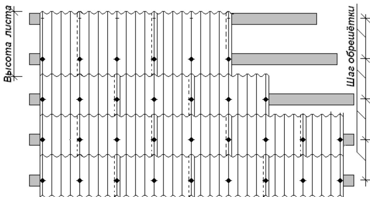
Рисунок 1. Схема монтажа и точки крепления черепицы Керамопласт при укладке со смещением, «зигзагом».
